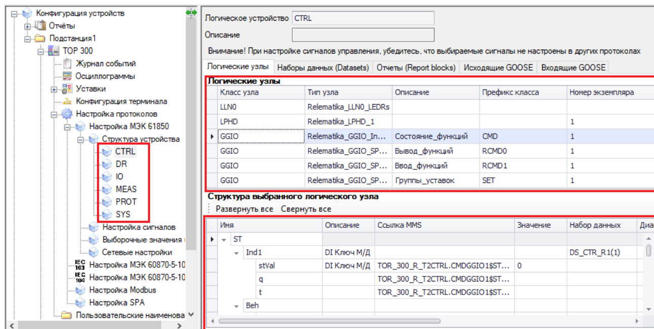
Рисунок 5.76 – Структура МЭК 61850
