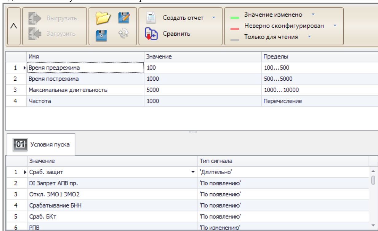
Рисунок 5.37 – Область конфигурирования осциллографа
