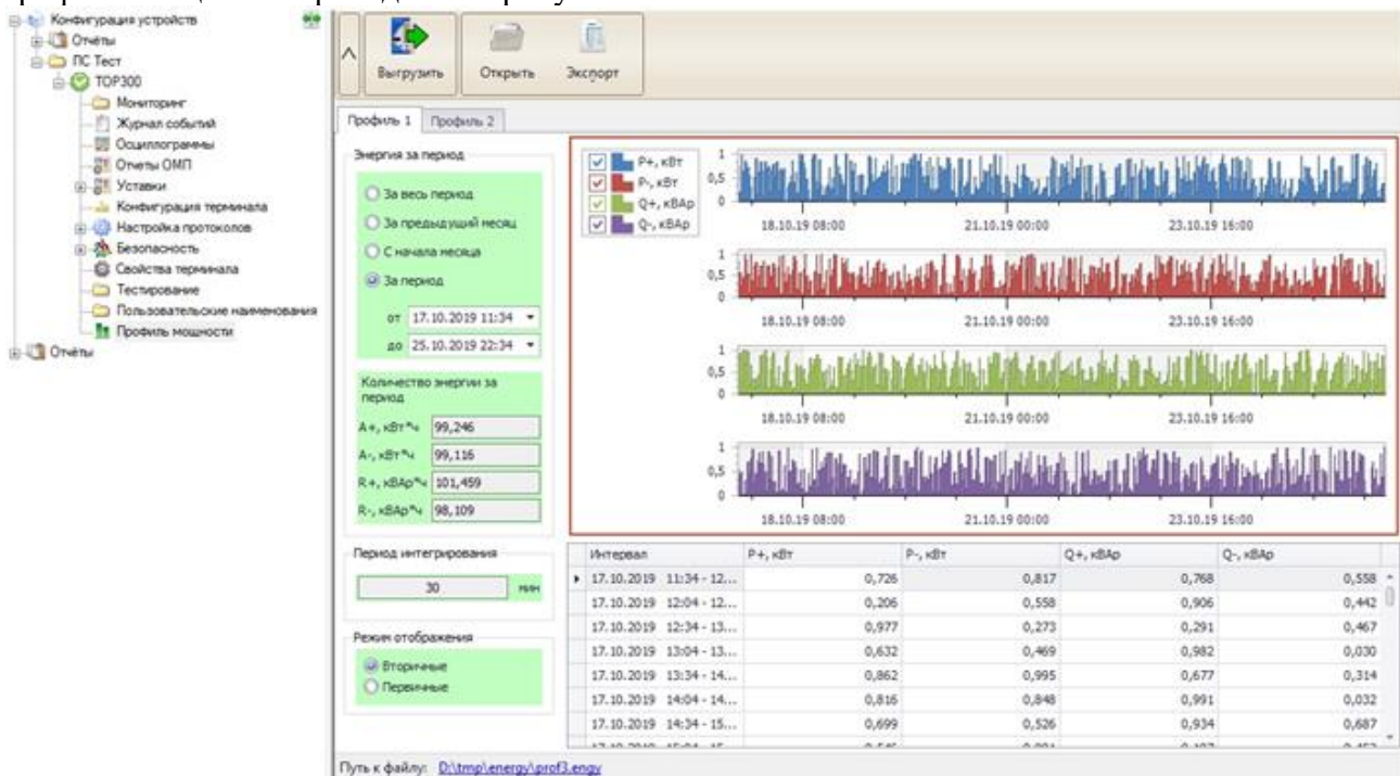
Рисунок 5.102 – Профиль мощности
