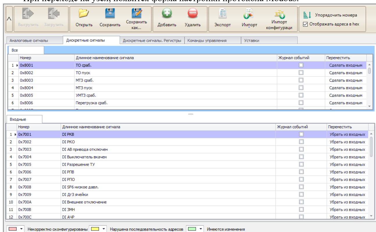
Рисунок 5.69 – Настройка Modbus
